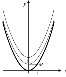
Рис. 2. Интегральные кривые уравнения
