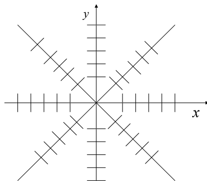
Рис. 4. Изоклины и поле направлений
